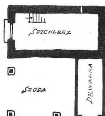
RZUT ŚPICHLERZA.
