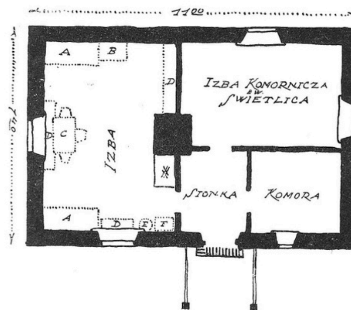
RZUT CHATY.
