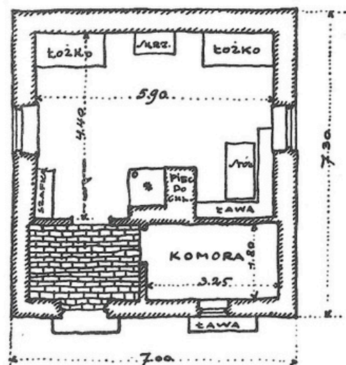
RZUT CHATY.
