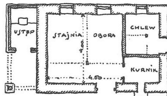
RZUT BUDYNKU DLA INWENTARZA.
