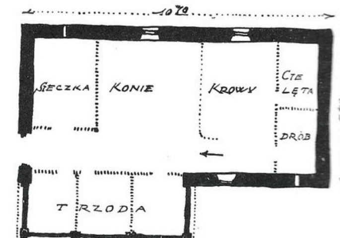
RZUT BUDYNKU DLA INWENTARZA.
